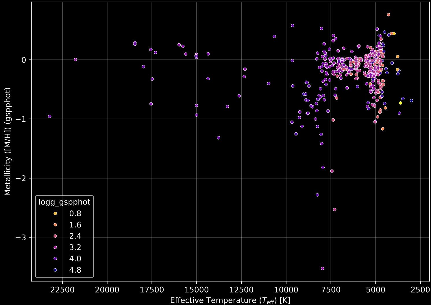
APOGEE DR17 Field: [120+00] Stellar Population Parameters (n= 440)
